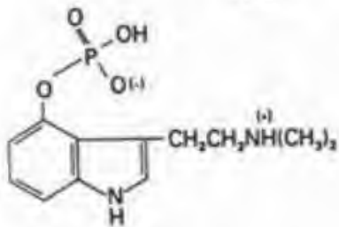
PSILOCYBIN
